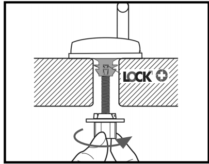
STEP 2 HINGE FIT
