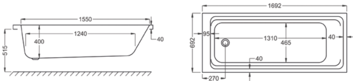
Tarn 1700 x 700mm
