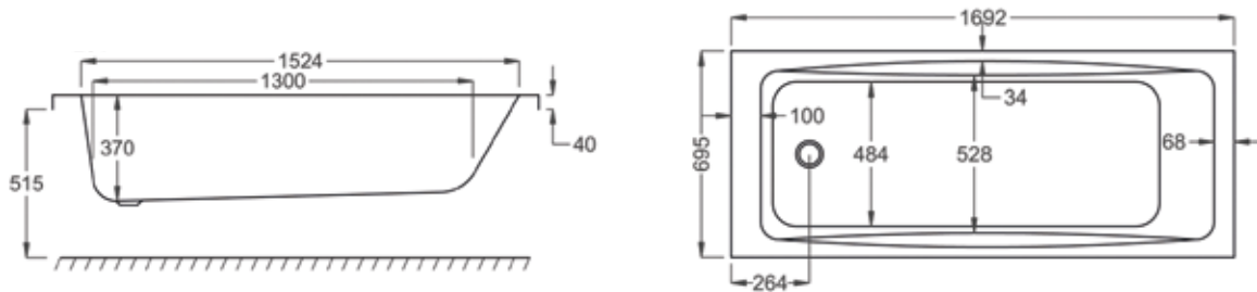
Burgos 1700 x 700mm
