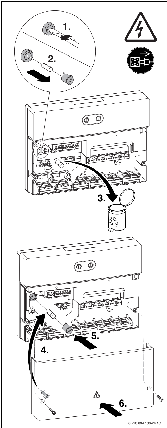
Fig. 25 Replace fuse
