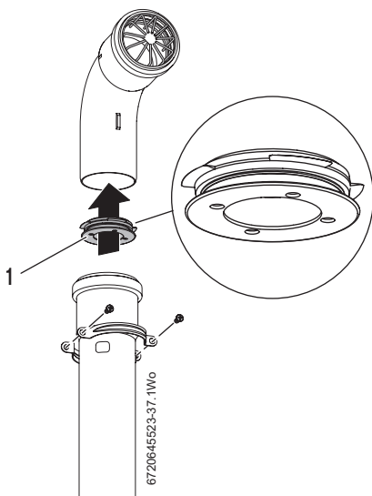
Fig. 42 Flue damper
