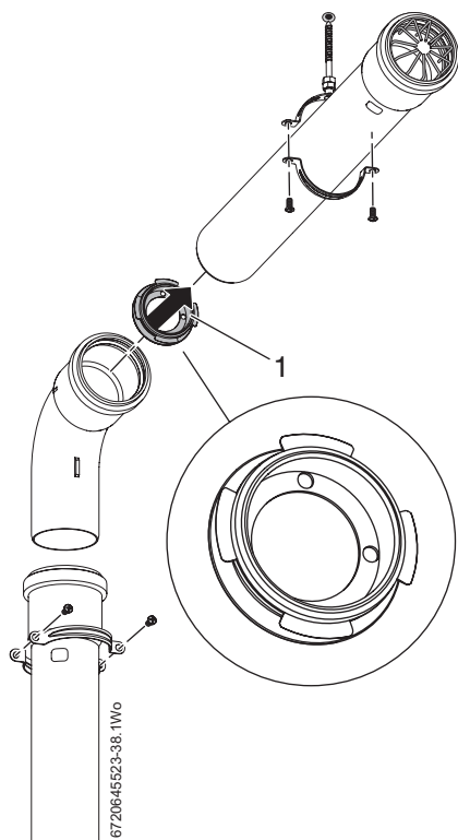
Fig. 49 Flue damper
